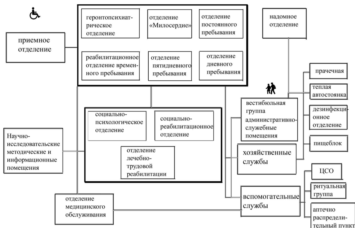
Рис. 1. Функциональные связи групп помещений геронтологического центра.
