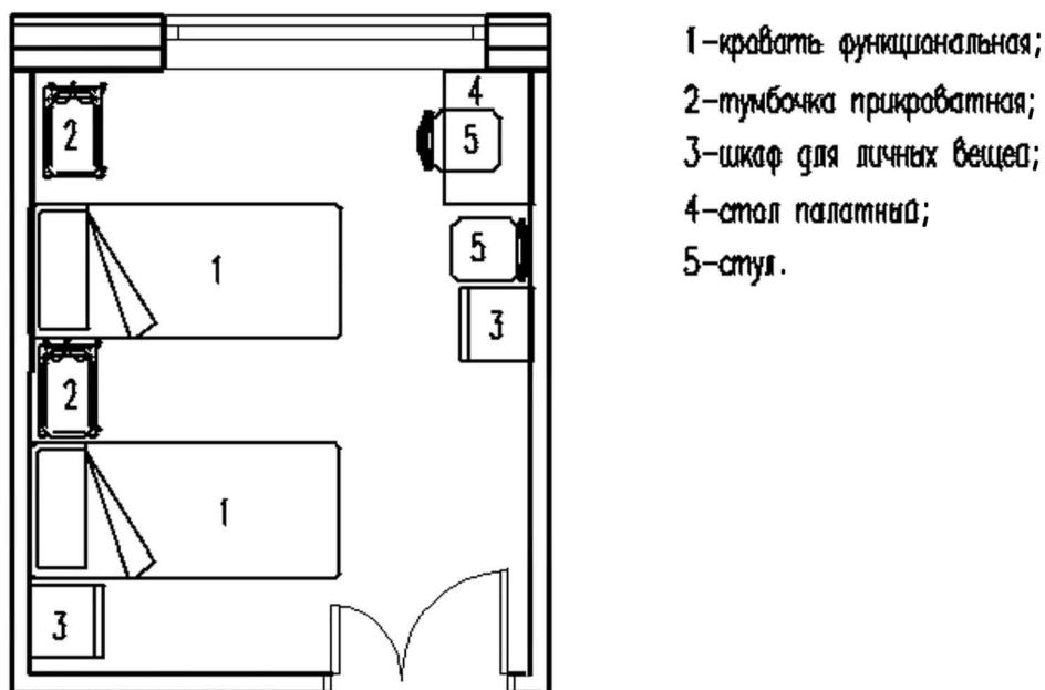
Рис. 4. Палата на 2 койки.
