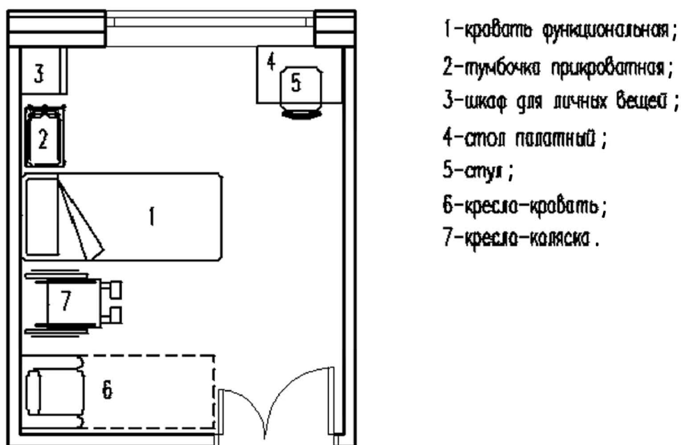
Рис. 3. Палата на 1 койку с местом отдыха сопровождающего.
